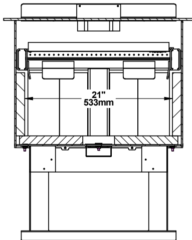
Chambre à combustion - Vue de face
