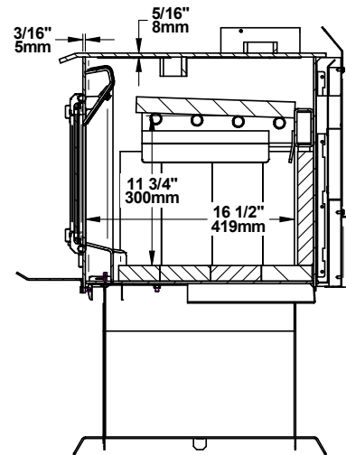
Chambre à combustion - Vue de côté
